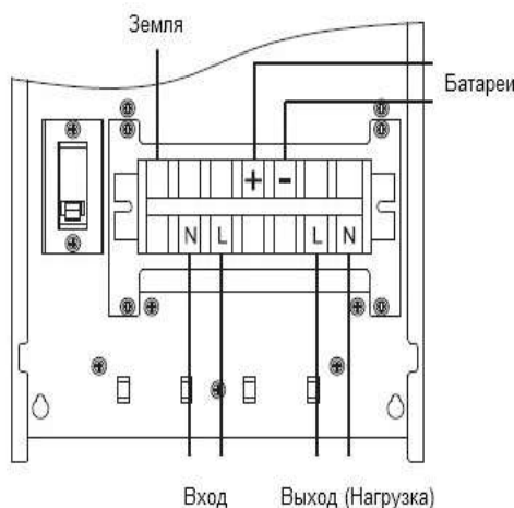
Схема подключения для моделей 6кВА и 10кВА
