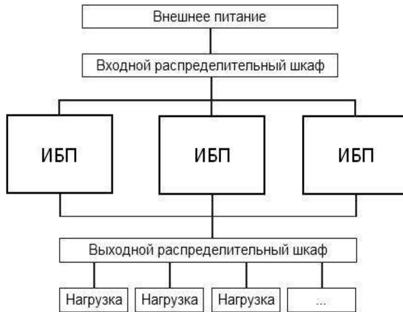
Структурная схема параллельной системы
