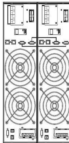
Параллельная система из двух ИБП
