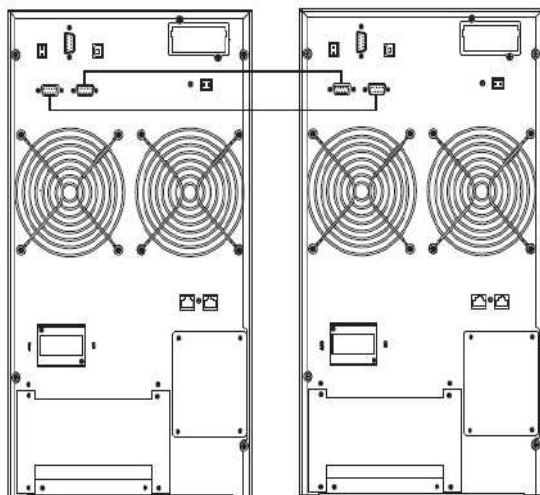
Параллельная система из двух ИБП
