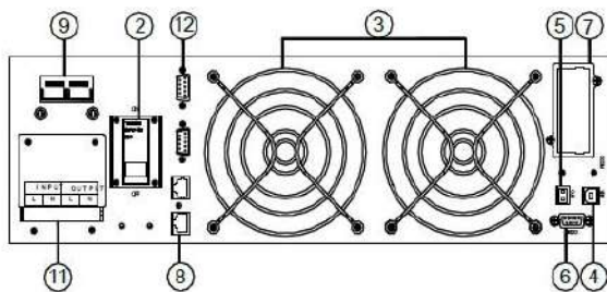
ИБП 6кВа и 10кВа
